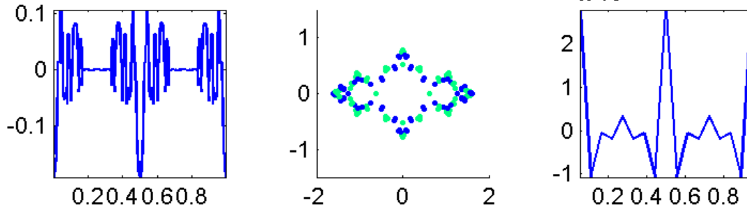
Num48 Eigval13491.3946
