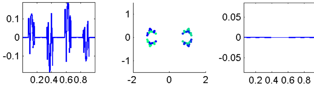
Num46 Eigval13320.9198+6.68339383e-012i
