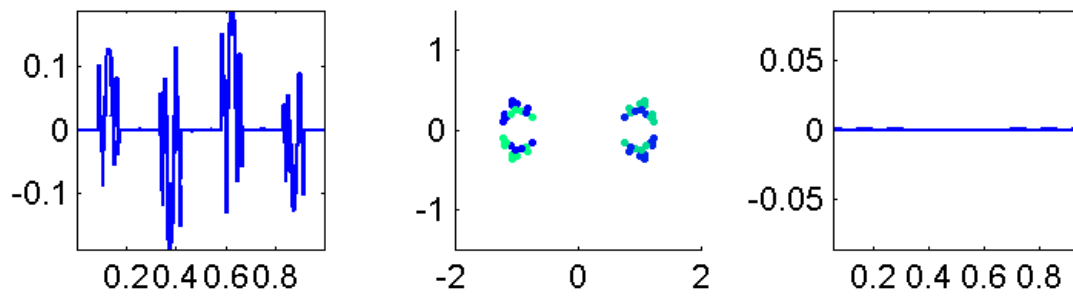
Num47 Eigval13491.392
