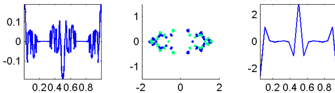
Num48 Eigval13491.3946
