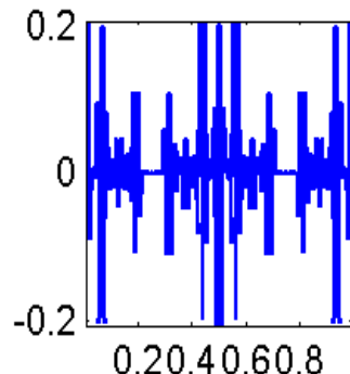
Num75
