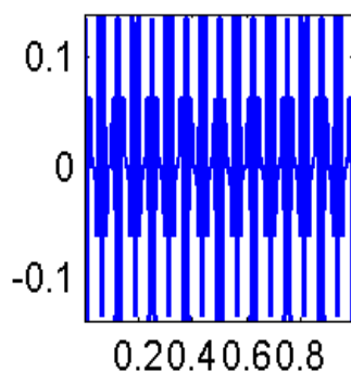
Num76
