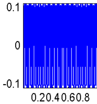
Num66
