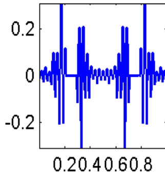
Num44
