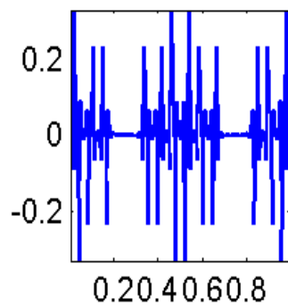
Num99
