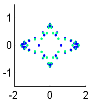
Eigval30665.6347
