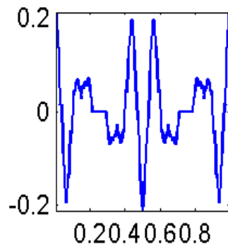
Num11
