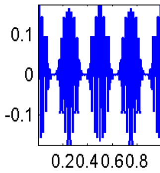
Num68
