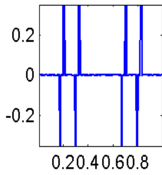
Num55
