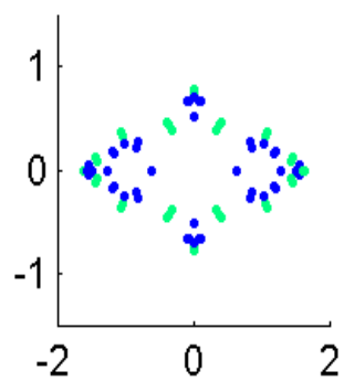
Eigval2806.1969
