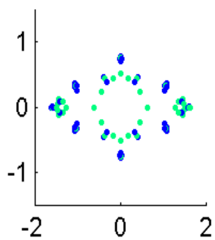
Eigval33660.8501
