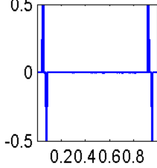
Num56
