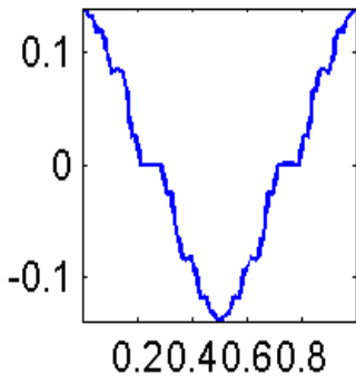
Num3
