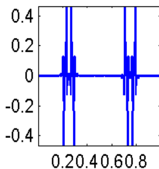
Num100
