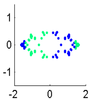
Eigval316.6279
