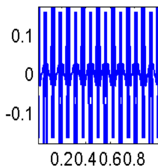
Num119
