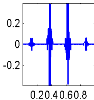
Num72
