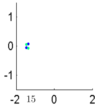
Eigval8688.9281
