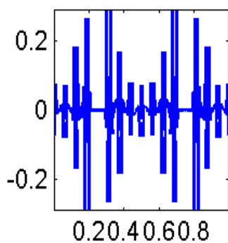
Num118
