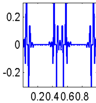
Num48
