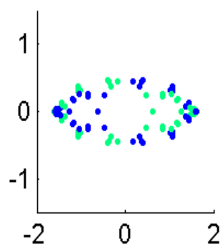
Eigval2391.4028
