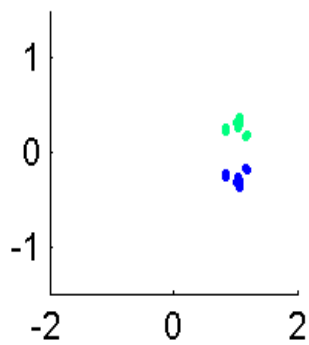
Eigval546.8995
