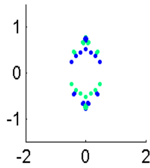
Eigval6593.633
