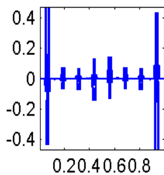
Num115
