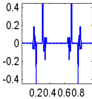
Num54
