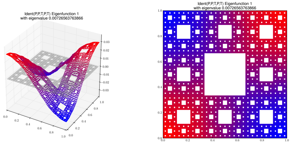
Eigenfunction 1 with eigenvalue 0.00726563763866
