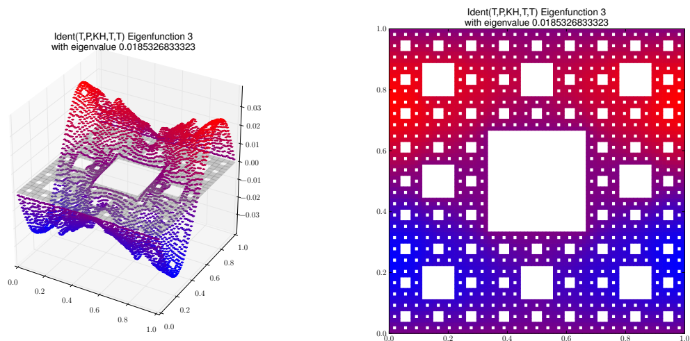
Eigenfunction 3 with eigenvalue 0.0185326833323
