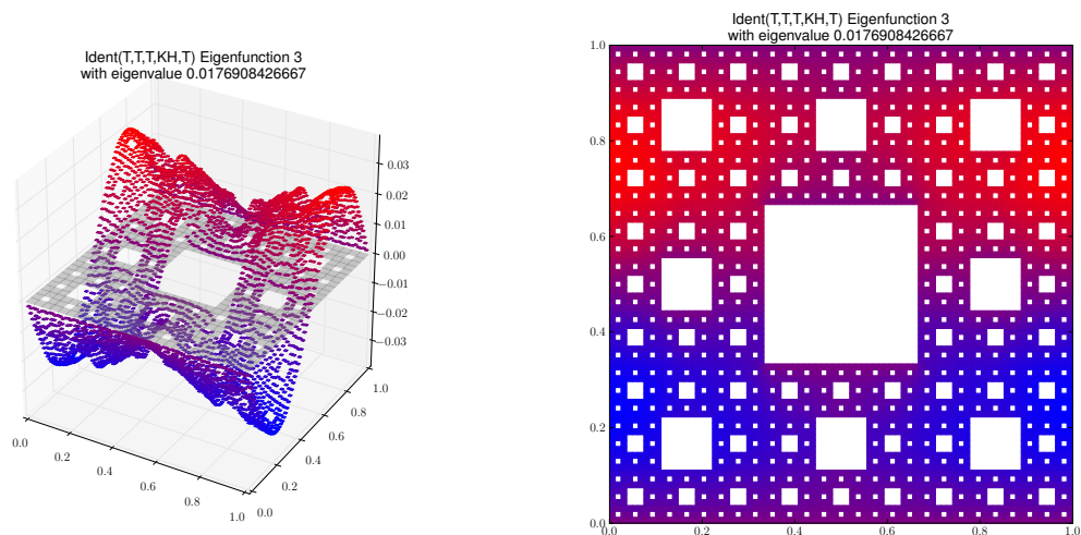
Eigenfunction 3 with eigenvalue 0.0176908426667
