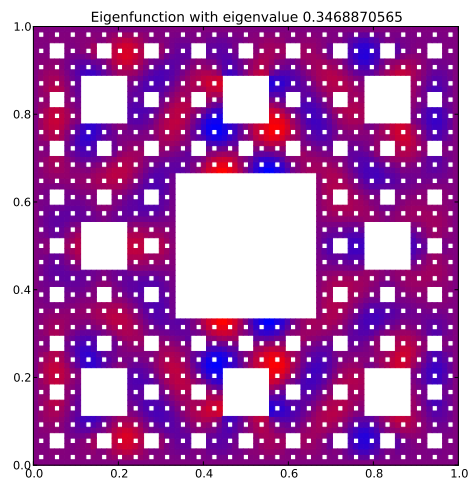
Eigenfunction 73 with eigenvalue 0.3468870565
