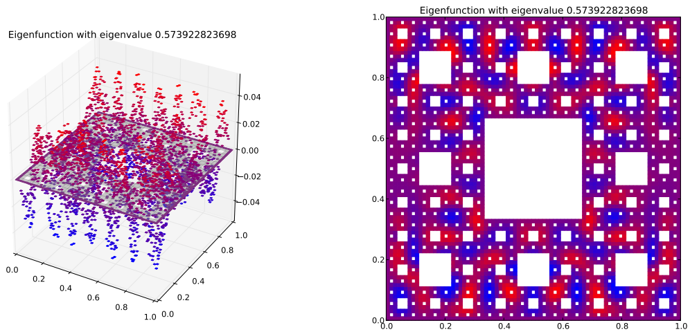
Eigenfunction 135 with eigenvalue 0.573922823698
