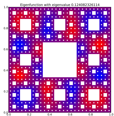
Eigenfunction 18 with eigenvalue 0.124082326114
