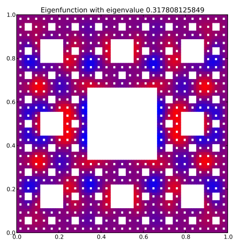
Eigenfunction 66 with eigenvalue 0.317808125849
