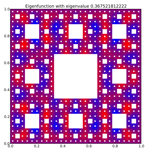
Eigenfunction 78 with eigenvalue 0.367521812222
