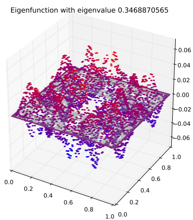
Eigenfunction 73 with eigenvalue 0.3468870565
