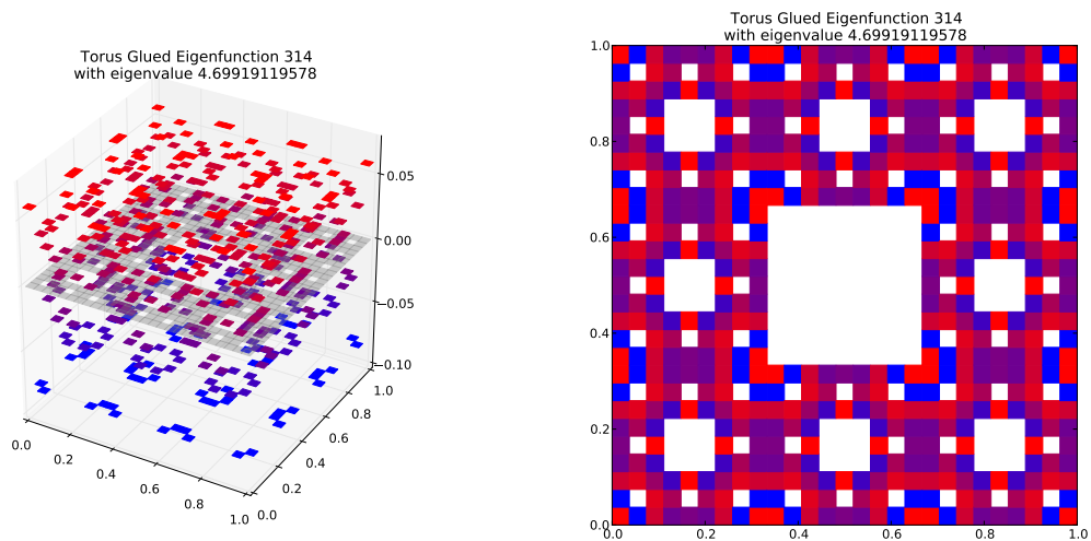
Eigenfunction 314 with eigenvalue 4.69919119578
