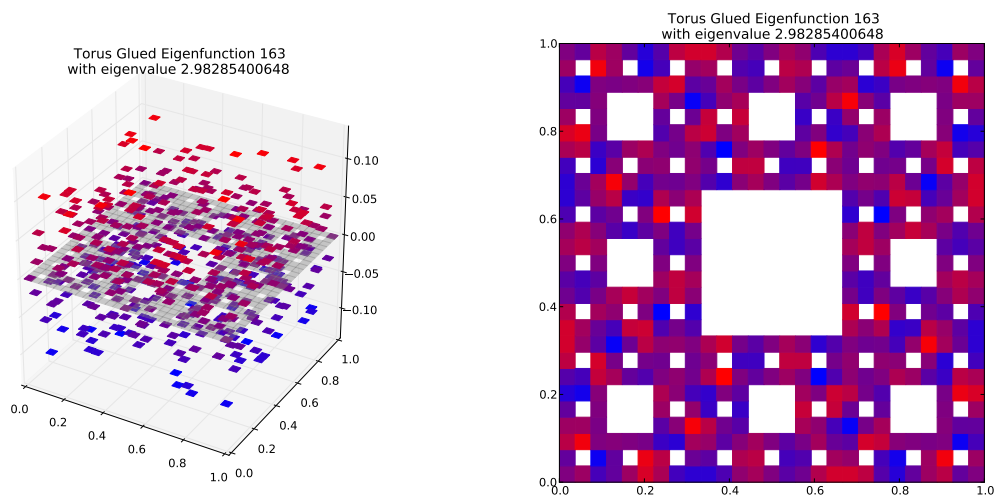
Eigenfunction 163 with eigenvalue 2.98285400648
