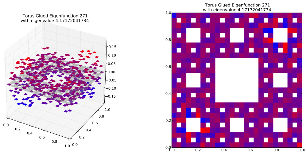
Eigenfunction 271 with eigenvalue 4.17172041734
