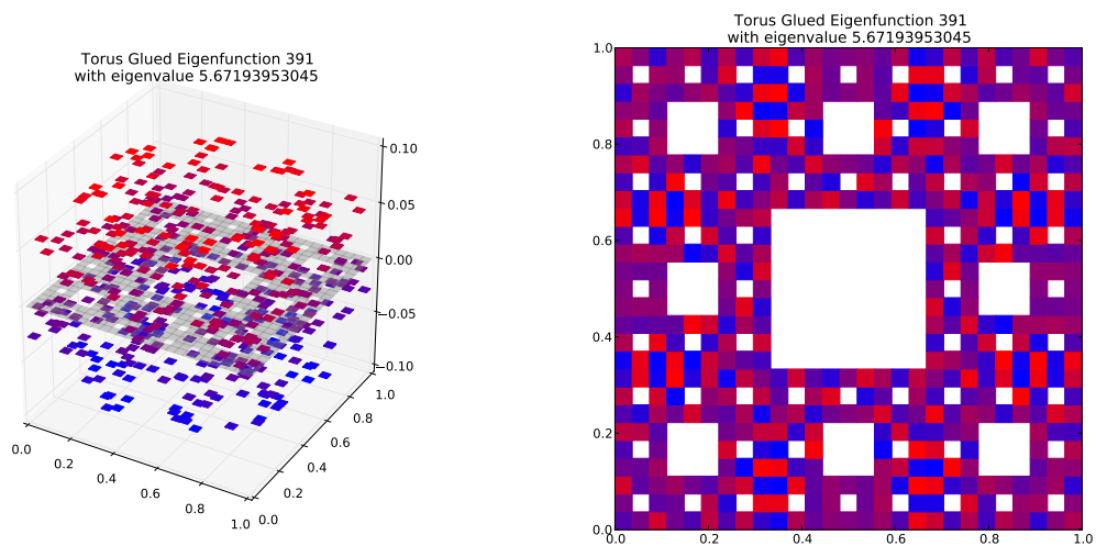
Eigenfunction 391 with eigenvalue 5.67193953045
