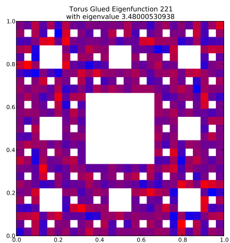
Eigenfunction 221 with eigenvalue 3.48000530938
