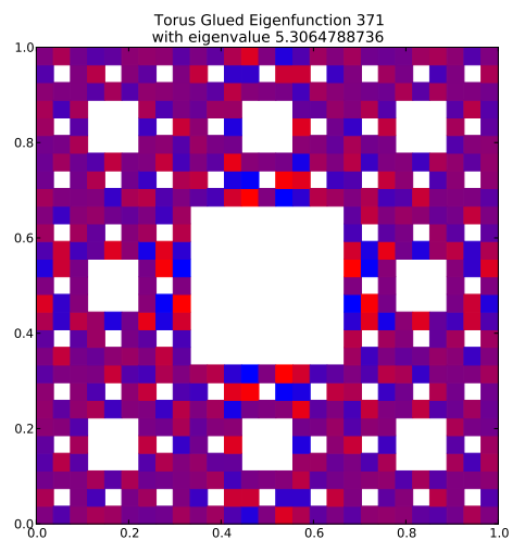
Eigenfunction 371 with eigenvalue 5.3064788736
