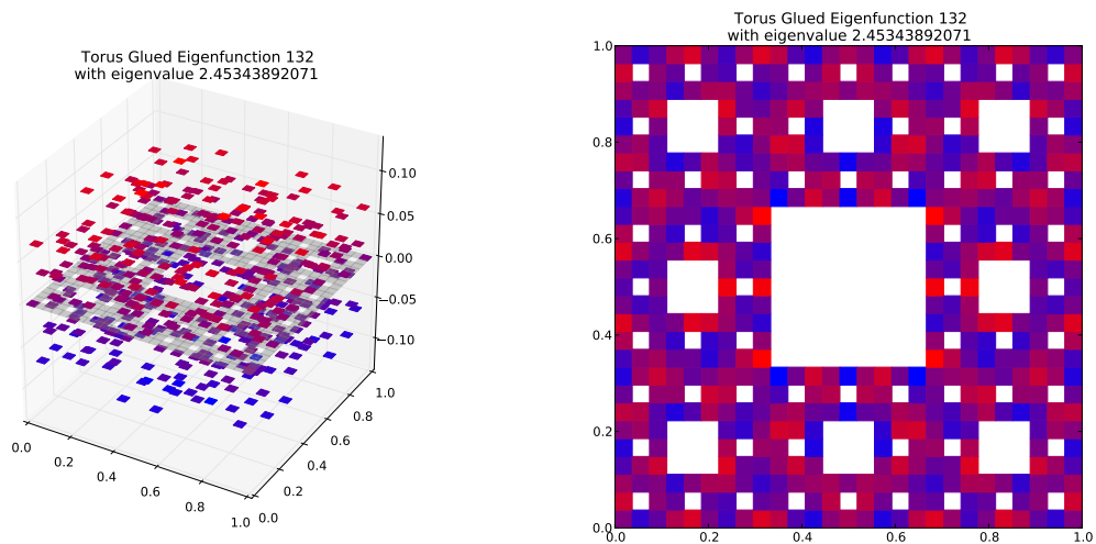
Eigenfunction 132 with eigenvalue 2.45343892071
