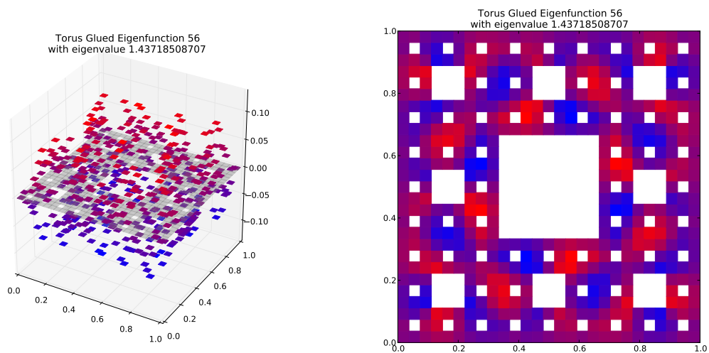
Eigenfunction 56 with eigenvalue 1.43718508707
