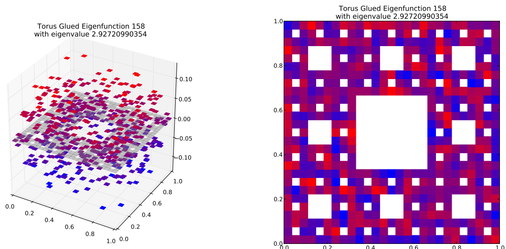
Eigenfunction 158 with eigenvalue 2.92720990354
