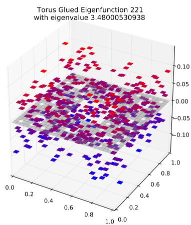
Eigenfunction 221 with eigenvalue 3.48000530938
