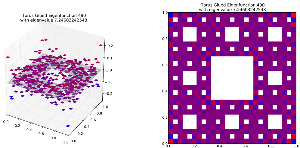
Eigenfunction 490 with eigenvalue 7.24603242548
