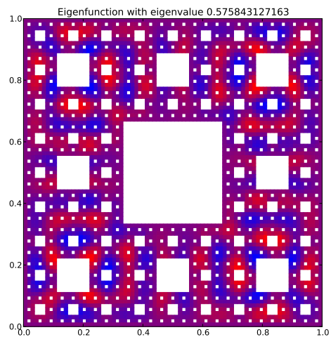
Eigenfunction 135 with eigenvalue 0.575843127163
