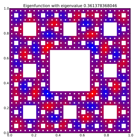
Eigenfunction 76 with eigenvalue 0.361378368046
