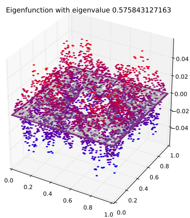
Eigenfunction 135 with eigenvalue 0.575843127163
