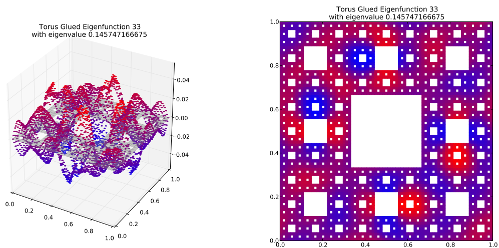
Eigenfunction 33 with eigenvalue 0.145747166675
