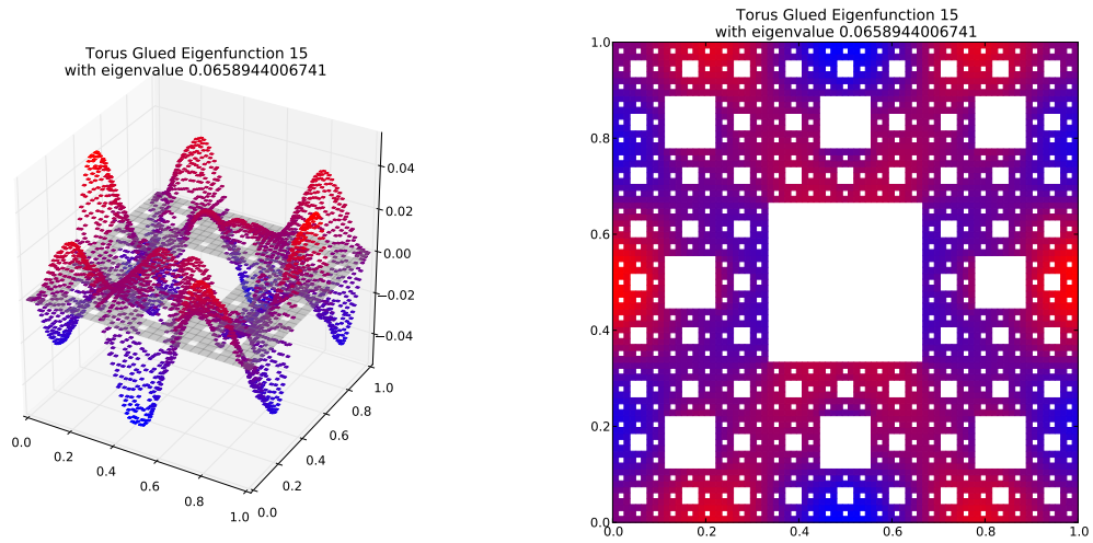
Eigenfunction 15 with eigenvalue 0.0658944006741
