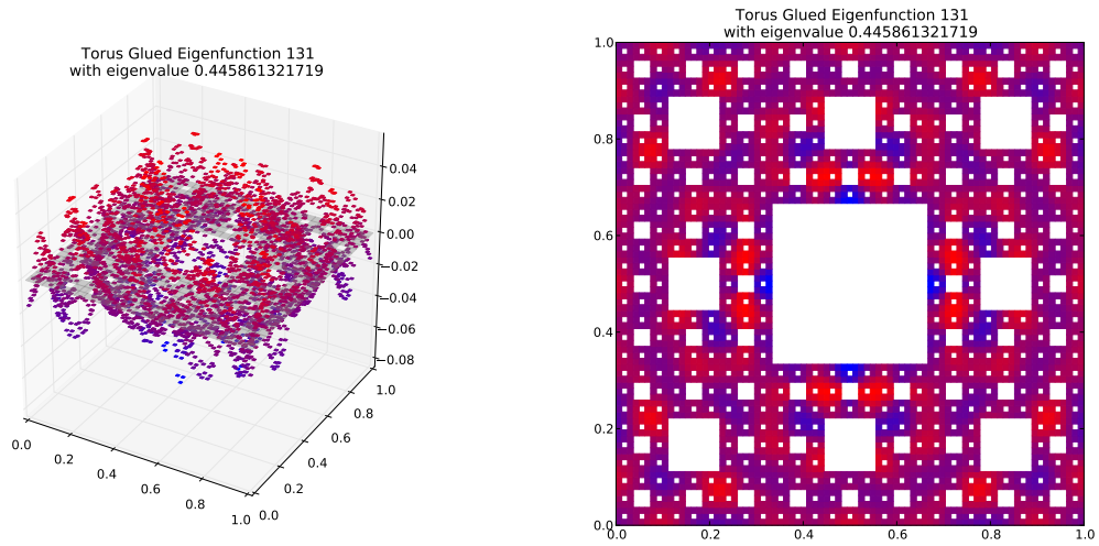
Eigenfunction 131 with eigenvalue 0.445861321719
