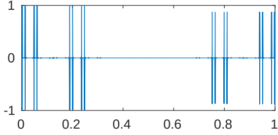
m=5 p=0.01 \lambda_{817}=42963228284745.11
