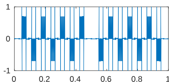
m=5 p=0.001 \lambda_{558}=2.059009415208845\text{e}+18
