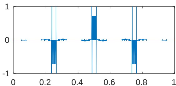
m=5 p=0.001 \lambda_{533}=2.05898969145559\text{e}+18
