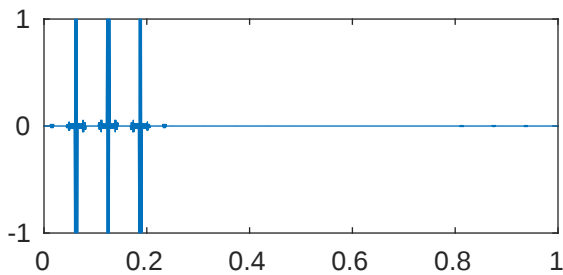
m=5 p=0.001 \lambda_{877}=4.116015886443784\text{e+18}
