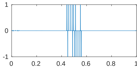
m=5 p=1e-05 \lambda_{656}=2.05268209929345\text{e}+28
