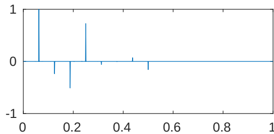
m=5 p=1e-05 \lambda_{614}=2.052676969698152\text{e}+28
