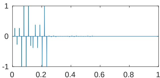
m=5 p=1e-05 \lambda_{437}=2.043529965232507\text{e}+28
