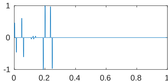
m=5 p=1e-05 \lambda_{242}=1.024053761598605\text{e}+23
