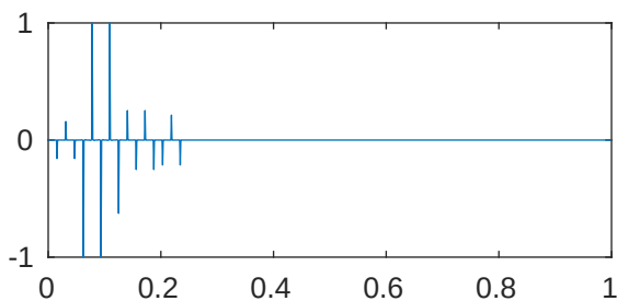
m=5 p=1e-05 \lambda_{323}=2.043515482907638\text{e}+28
