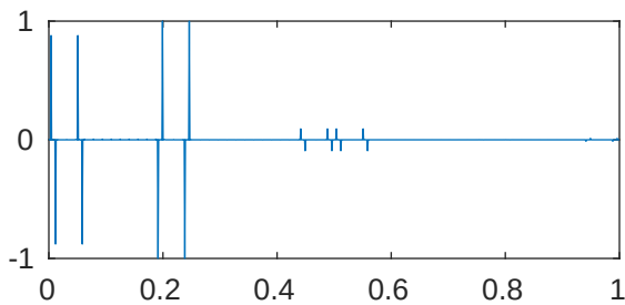
m=5 p=1e-05 \lambda_{643}=2.052682087872147\text{e}+28
