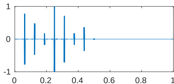
m=5 p=1e-05 \lambda_{940}=4.096199697451703\text{e}+28
