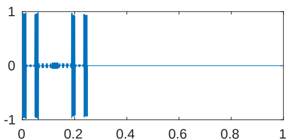
m=5 p=1e-05 \lambda_{893}=4.096199685945233\text{e}+28
