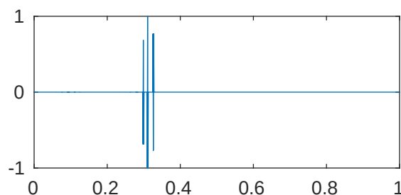
m=5 p=1e-05 \lambda_{816}=4.096194565675239\text{e}+28
