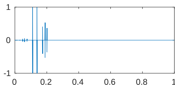
m=5 p=1e-05 \lambda_{792}=4.096194565656553\text{e}+28
