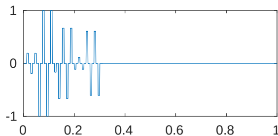
m=5 p=1e-05 \lambda_{190}=5.136428593182933\text{e}+22
