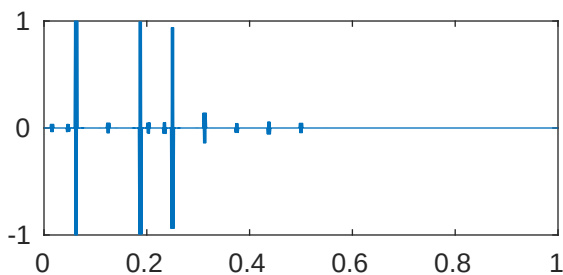
m=5 p=1e-05 \lambda_{861}=4.096199674509041\text{e}+28
