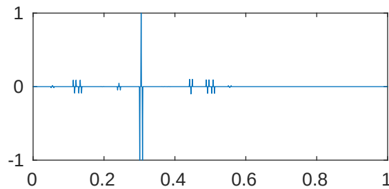
m=5 p=1e-05 \lambda_{314}=2.04162574271622\text{e}+28
