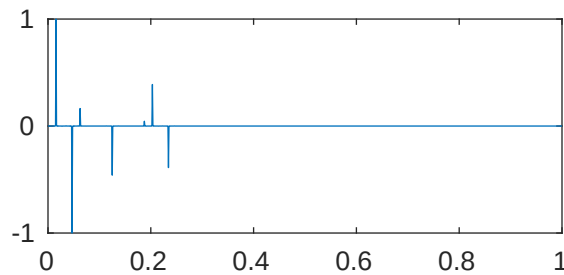
m=5 p=1e-05 \lambda_{416}=2.043527841463583\text{e}+28
