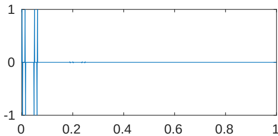
m=5 p=1e-05 \lambda_{499}=2.048102386895015\text{e}+28
