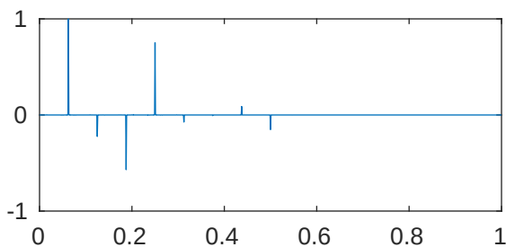
m=5 p=1e-05 \lambda_{423}=2.043527846439715\text{e}+28
