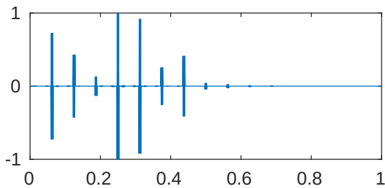
m=5 p=1e-05 \lambda_{877}=4.096199674556642\text{e}+28
