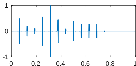
m=5 p=1e-05 \lambda_{942}=4.096199697462515\text{e}+28
