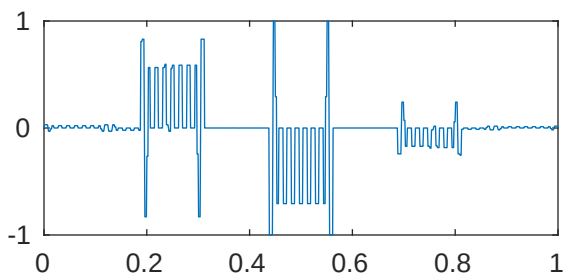
m=5 p=1e-05 \lambda_{135}=5.120254907467739\text{e}+22
