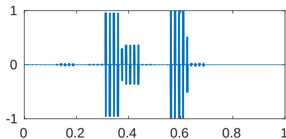
m=5 p=1e-05 \lambda_{846}=4.096199669799314\text{e}+28
