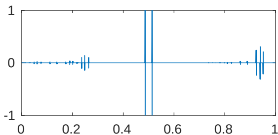
m=5 p=1e-05 \lambda_{795}=4.096194565656624\text{e}+28
