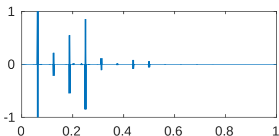
m=5 p=1e-05 \lambda_{863}=4.096199674514499\text{e}+28
