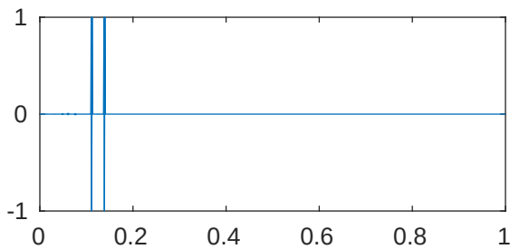
m=5 p=1e-05 \lambda_{793}=4.096194565656556\text{e}+28
