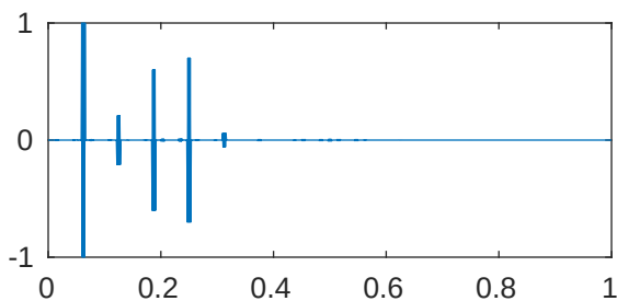
m=5 p=1e-05 \lambda_{933}=4.096199697421729\text{e}+28
