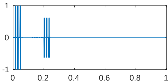
m=5 p=1e-05 \lambda_{835}=4.096199669762611\text{e}+28
