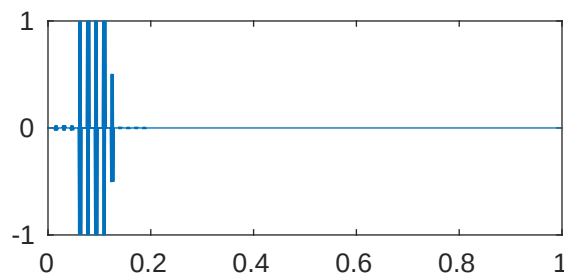
m=5 p=1e-05 \lambda_{954}=4.096199702164847\text{e}+28
