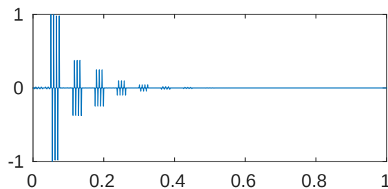
m=5 p=1e-05 \lambda_{292}=2.041625738678072\text{e}+28
