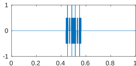
m=5 p=1e-05 \lambda_{910}=4.096199685988862\text{e}+28
