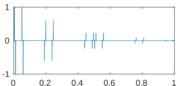
m=5 p=1e-05 \lambda_{641}=2.052682087859845\text{e}+28
