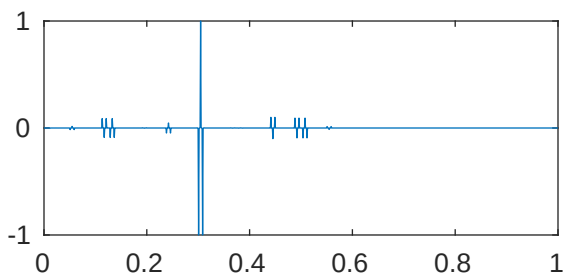
m=5 p=1e-05 \lambda_{315}=2.04162574271622\text{e}+28
