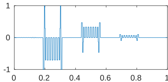
m=5 p=1e-05 \lambda_{134}=5.120254896607353\text{e}+22
