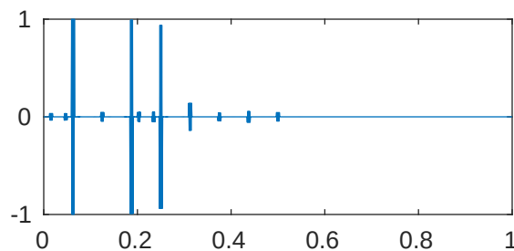
m=5 p=1e-05 \lambda_{862}=4.096199674509041\text{e}+28
