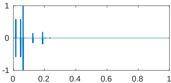
m=5 p=1e-05 \lambda_{859}=4.09619967450514\text{e}+28
