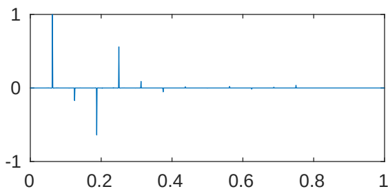
m=5 p=1e-05 \lambda_{357}=2.043517605630193\text{e}+28
