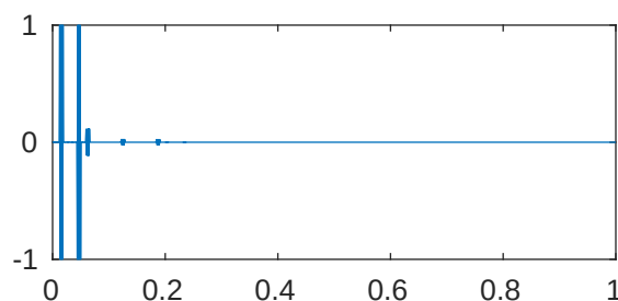
m=5 p=1e-05 \lambda_{858}=4.096199674504755\text{e}+28
