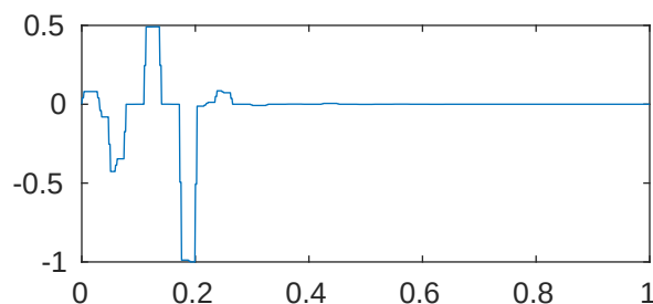
m=5 p=1e-05 \lambda_{24}=1.279441549702985\text{e}+17
