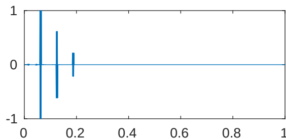
m=5 p=1e-05 \lambda_{852}=4.096199674495909\text{e}+28
