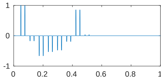
m=5 p=1e-05 \lambda_{218}=1.024052481442647\text{e}+23
