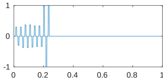
m=5 p=1e-05 \lambda_{182}=5.136428498557179\text{e}+22
