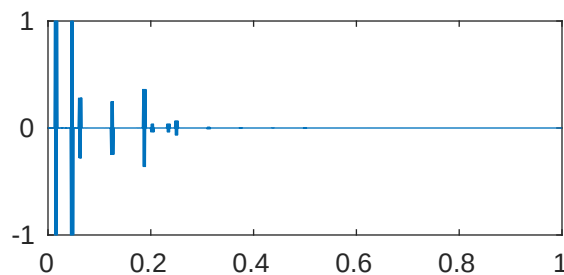
m=5 p=1e-05 \lambda_{856}=4.096199674504643\text{e}+28
