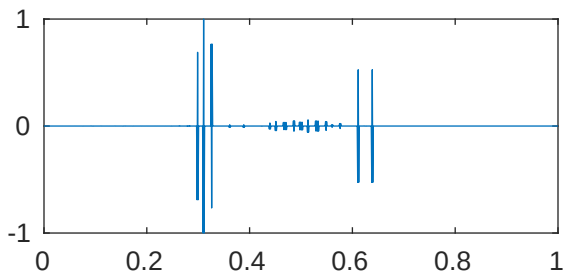
m=5 p=1e-05 \lambda_{817}=4.09619456567524\text{e}+28
