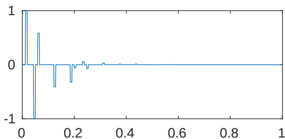
m=5 p=1e-05 \lambda_{159}=5.131685981456426\text{e}+22
