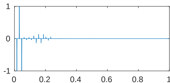
m=5 p=1e-05 \lambda_{330}=2.043515482914683\text{e}+28
