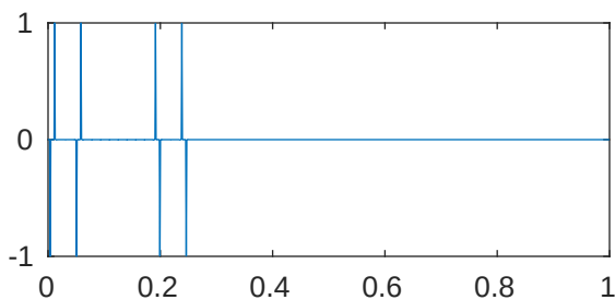
m=5 p=1e-05 \lambda_{381}=2.043522718311722\text{e}+28
