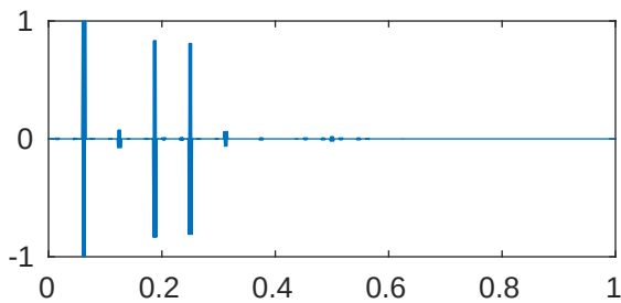
m=5 p=1e-05 \lambda_{871}=4.096199674523451\text{e}+28
