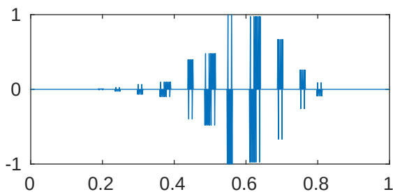
m=5 p=1e-05 \lambda_{575}=2.048112643567256\text{e}+28
