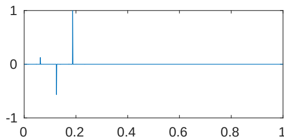
m=5 p=1e-05 \lambda_{364}=2.043517608414537\text{e}+28
