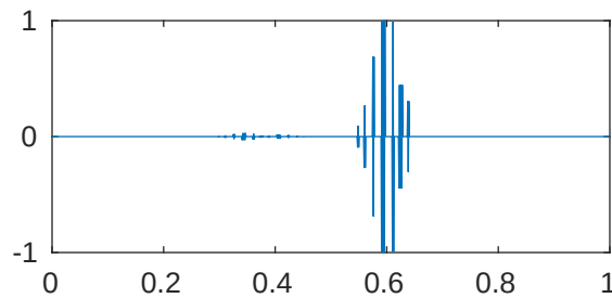
m=5 p=1e-05 \lambda_{830}=4.096194565693929\text{e}+28
