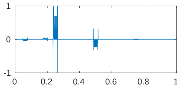
m=5 p=1e-05 \lambda_{472}=2.04809515391893\text{e}+28
