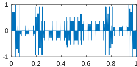
m=5 p=1e-05 \lambda_{542}=2.048109644172934\text{e}+28
