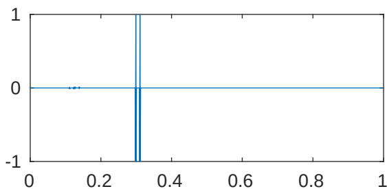
m=5 p=1e-05 \lambda_{809}=4.096194565669416\text{e}+28
