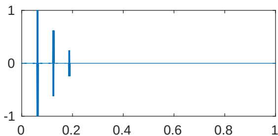
m=5 p=1e-05 \lambda_{873}=4.096199674532362\text{e}+28
