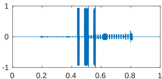
m=5 p=1e-05 \lambda_{897}=4.096199685963825\text{e}+28
