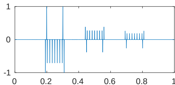
m=5 p=1e-05 \lambda_{646}=2.052682095926323\text{e}+28
