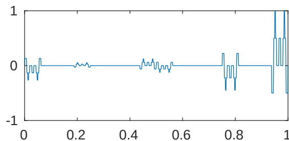
m=5 p=1e-05 \lambda_{112}=5.12021120396157\text{e}+22
