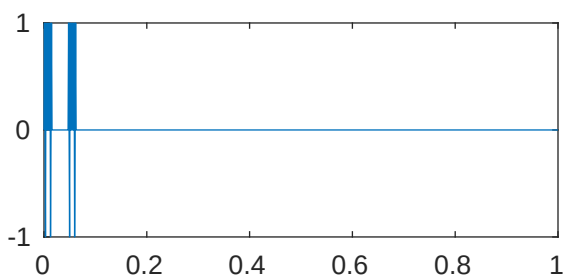
m=5 p=1e-05 \lambda_{563}=2.048112643542232\text{e}+28
