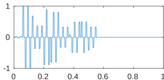
m=5 p=1e-05 \lambda_{180}=5.136428452778607\text{e}+22
