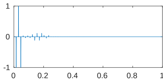
m=5 p=1e-05 \lambda_{586}=2.052674840963116\text{e}+28
