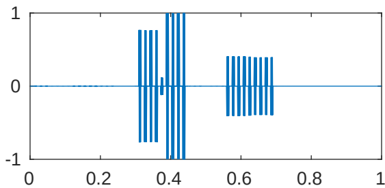
m=5 p=1e-05 \lambda_{847}=4.096199669799488\text{e}+28
