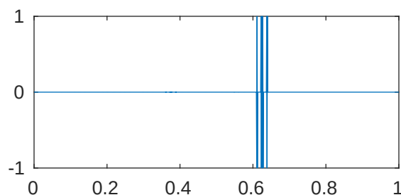
m=5 p=1e-05 \lambda_{804}=4.09619456566243\text{e}+28
