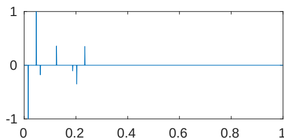
m=5 p=1e-05 \lambda_{606}=2.052676964718525\text{e}+28
