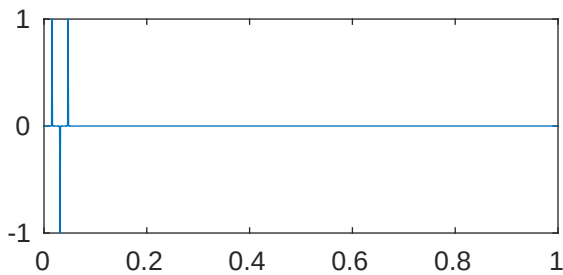
m=5 p=1e-05 \lambda_{433}=2.043529965220322\text{e}+28
