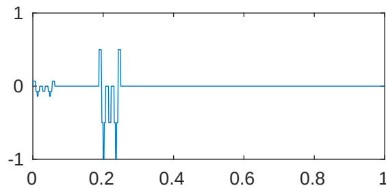
m=5 p=1e-05 \lambda_{116}=5.120211207702977\text{e}+22
