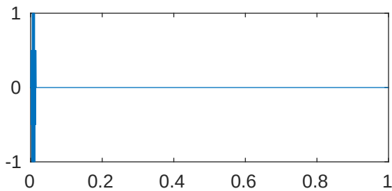
m=5 p=1e-05 \lambda_{967}=4.096204806155972\text{e}+28
