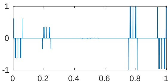
m=5 p=1e-05 \lambda_{627}=2.052682076385756\text{e}+28
