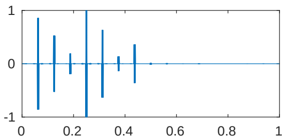
m=5 p=1e-05 \lambda_{875}=4.096199674551832\text{e}+28
