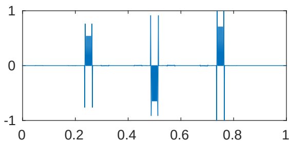
m=5 p=1e-05 \lambda_{491}=2.048095170154864\text{e}+28
