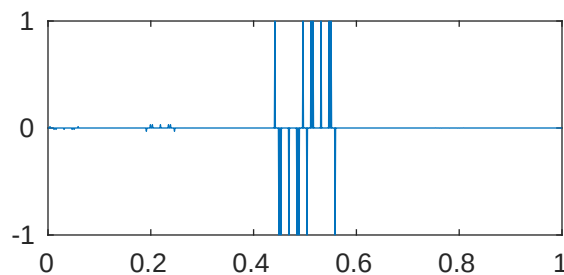
m=5 p=1e-05 \lambda_{628}=2.05268207639497\text{e}+28
