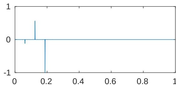
m=5 p=1e-05 \lambda_{660}=2.052687197795679\text{e}+28
