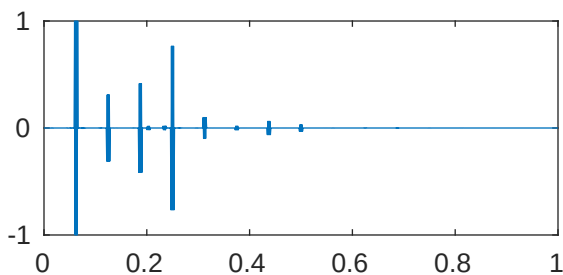
m=5 p=1e-05 \lambda_{927}=4.096199697412491\text{e}+28
