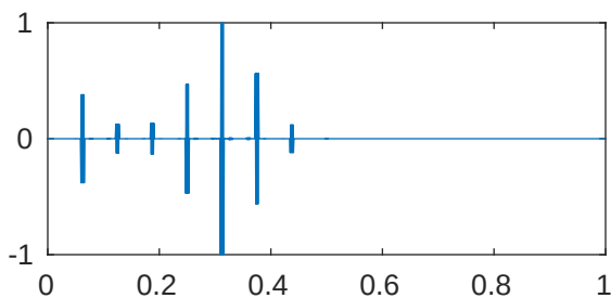
m=5 p=1e-05 \lambda_{879}=4.096199674568683\text{e}+28
