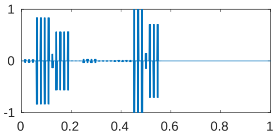
m=5 p=1e-05 \lambda_{841}=4.096199669780898\text{e}+28
