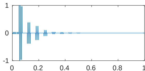
m=5 p=1e-05 \lambda_{288}=2.041625738673085\text{e}+28
