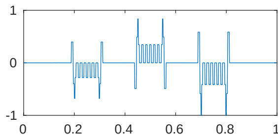
m=5 p=1e-05 \lambda_{118}=5.120218701950445\text{e}+22
