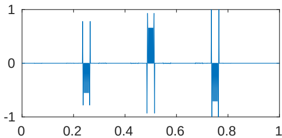
m=5 p=1e-05 \lambda_{469}=2.048095153883093\text{e}+28
