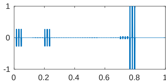
m=5 p=1e-05 \lambda_{946}=4.09619970214583\text{e}+28
