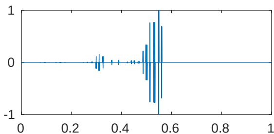
m=5 p=1e-05 \lambda_{813}=4.096194565675228\text{e}+28
