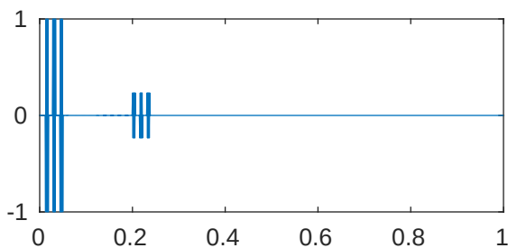
m=5 p=1e-05 \lambda_{945}=4.096199702145425\text{e}+28
