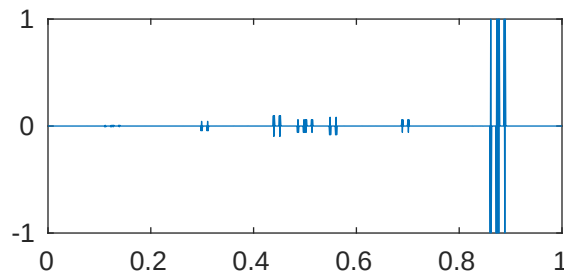
m=5 p=1e-05 \lambda_{812}=4.096194565669452\text{e}+28
