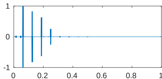
m=5 p=1e-05 \lambda_{850}=4.096199674495254\text{e}+28
