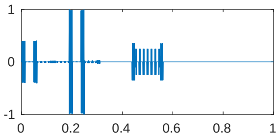
m=5 p=1e-05 \lambda_{889}=4.096199685945155\text{e}+28
