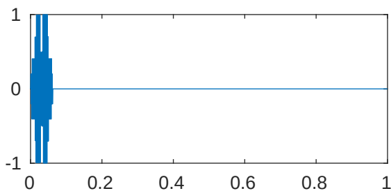
m=5 p=1e-05 \lambda_{983}=4.096204806187312\text{e}+28
