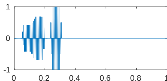
m=5 p=1e-05 \lambda_{762}=2.054579071579842\text{e}+28
