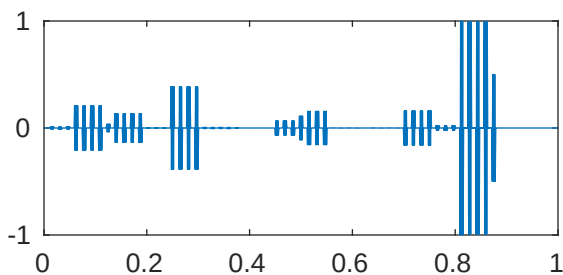
m=5 p=1e-05 \lambda_{837}=4.096199669780208\text{e}+28
