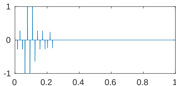
m=5 p=1e-05 \lambda_{324}=2.043515482907828\text{e}+28
