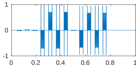
m=5 p=1e-05 \lambda_{532}=2.048109632732328\text{e}+28
