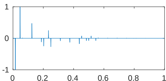
m=5 p=1e-05 \lambda_{605}=2.052676964710837\text{e}+28
