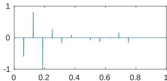
m=5 p=1e-05 \lambda_{402}=2.043527833300478\text{e}+28
