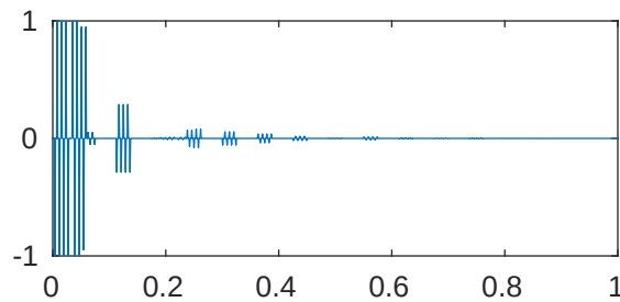
m=5 p=1e-05 \lambda_{284}=2.041625738668342\text{e}+28
