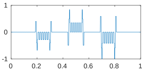
m=5 p=1e-05 \lambda_{119}=5.120218701950445\text{e}+22
