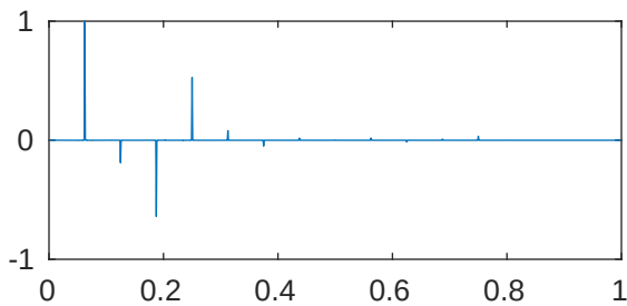
m=5 p=1e-05 \lambda_{421}=2.043527846222345\text{e}+28
