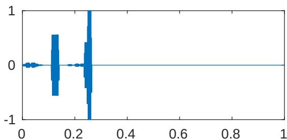
m=5 p=1e-05 \lambda_{987}=4.096204806187371\text{e}+28
