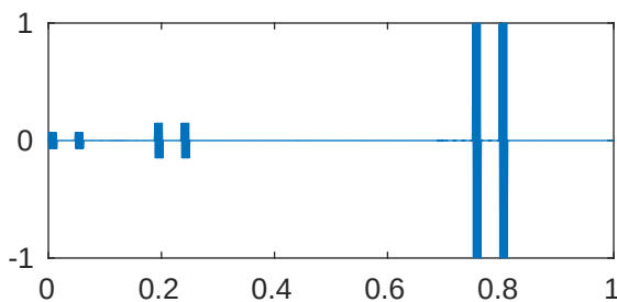
m=5 p=1e-05 \lambda_{885}=4.096199685944593\text{e}+28
