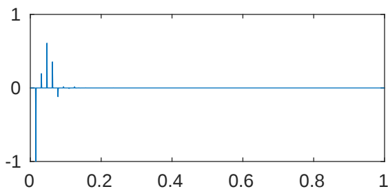
m=5 p=1e-08 \lambda_{383}=2.047855261194814\text{e}+43
