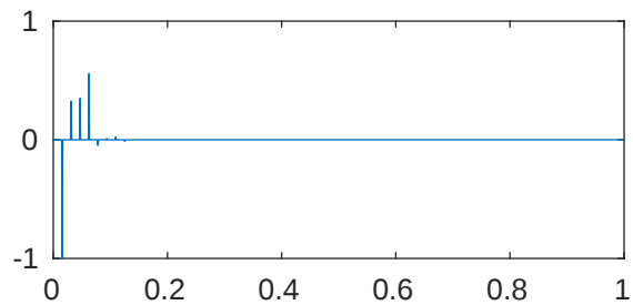
m=5 p=1e-08 \lambda_{368}=2.047855257996498\text{e}+43
