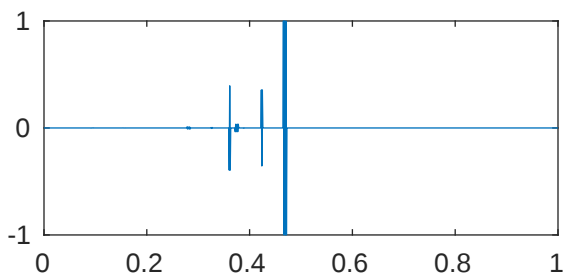
m=5 p=1e-08 \lambda_{857}=4.096000132815768\text{e}+43
