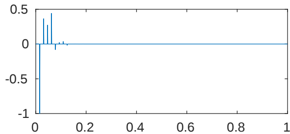
m=5 p=1e-08 \lambda_{367}=2.047855257180363\text{e}+43
