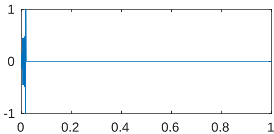
m=5 p=1e-08 \lambda_{997}=4.096000158517192e+43
