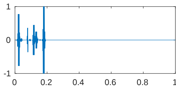
m=5 p=1e-08 \lambda_{894}=4.096000137935767\text{e}+43
