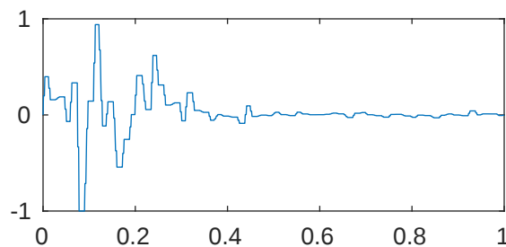
m=5 p=1e-08 \lambda_{54}=8.00514464729231e+27
