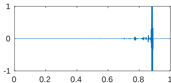
m=5 p=1e-08 \lambda_{880}=4.096000137935762\text{e}+43
