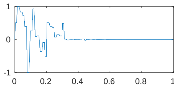
m=5 p=1e-08 \lambda_{42}=3.180478672189975e+27
