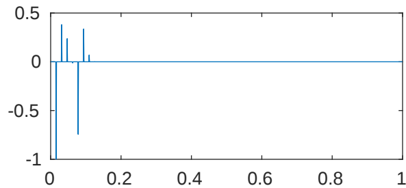
m=5 p=1e-08 \lambda_{362}=2.047855256167795\text{e}+43
