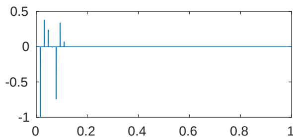
m=5 p=1e-08 \lambda_{363}=2.047855256167795\text{e}+43
