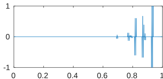
m=5 p=1e-08 \lambda_{312}=2.047795276674017\text{e}+43
