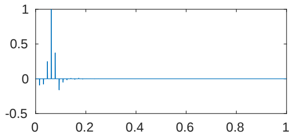
m=5 p=1e-08 \lambda_{369}=2.047855258043249\text{e}+43
