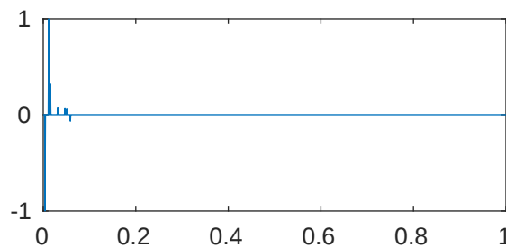
m=5 p=1e-08 \lambda_{432}=2.04785527148714\text{e}+43
