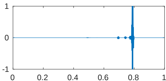
m=5 p=1e-08 \lambda_{933}=4.096000143055766e+43
