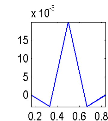
Eigval7317.6338
