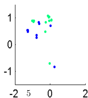
Eigval7317.6338
