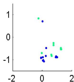
Eigval7317.6338
