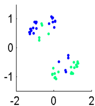
Eigval3264.9255
