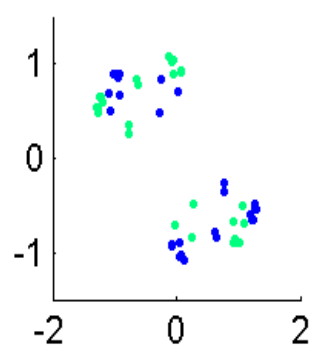
Eigval6603.1016
